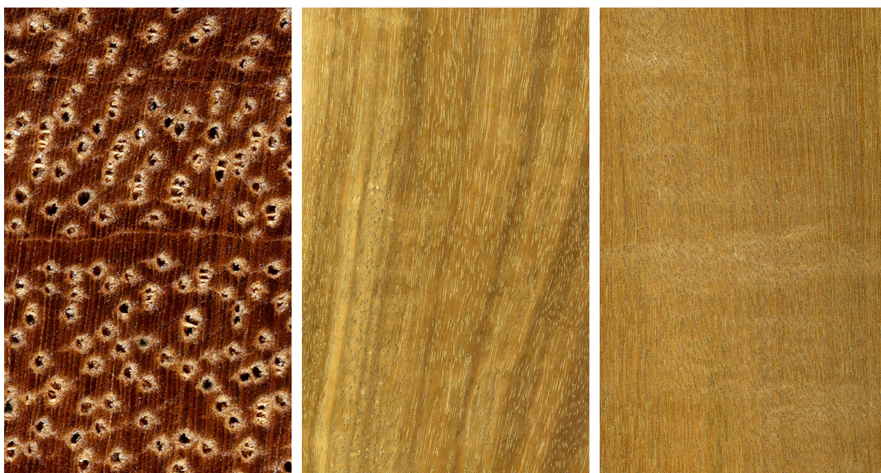
Tanimbuca ( Terminalia spp.): Querschnitt (ca. 10x); tangentielle und radiale Oberfläche (natürliche Größe)
