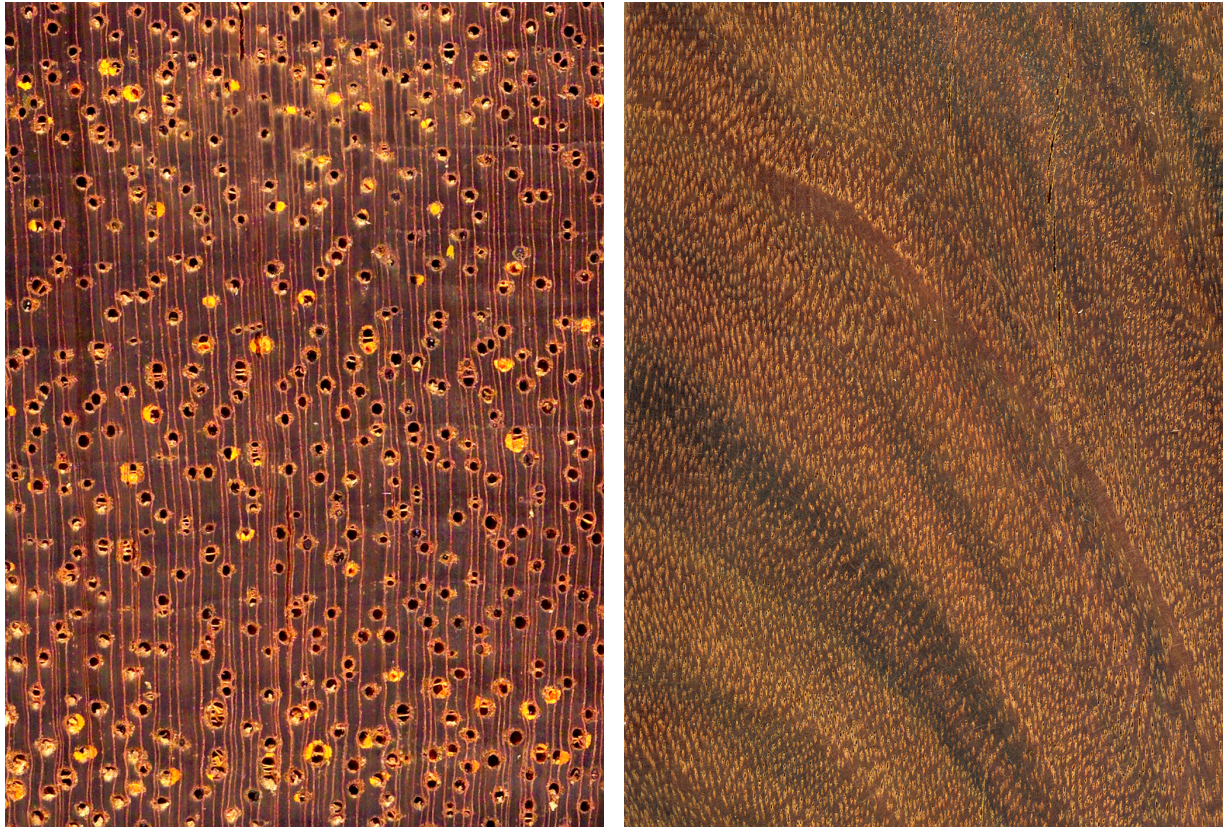
Okan ( Cylicodiscus gabonensis ): Querschnitt (ca. 12x) und tangentiale Oberfläche (natürliche Größe)
