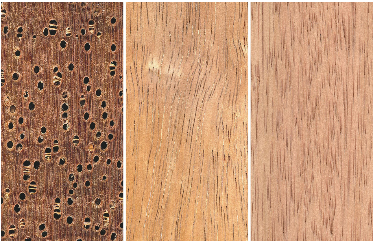
Cedrorana ( Cedrelinga cateniformis ): Querschnitt (ca. 12x) tangentiale und radiale Oberfläche (natürliche Größe)
