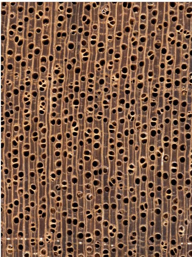
Gelbes Meranti ( Shorea spp.): Querschnitt (ca. 12x) und radiale Oberfläche (natürliche Größe)
